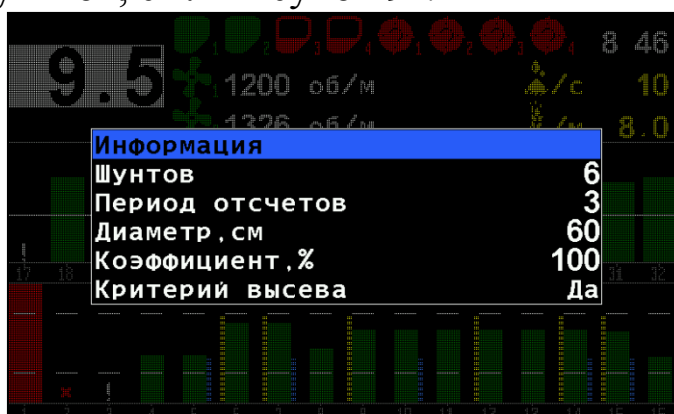
Рисунок 9 Параметры датчика скорости
