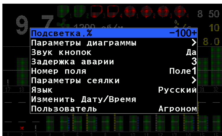
Рисунок 13 Меню настроек
