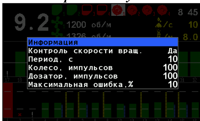
Рисунок 8 Параметры дозатора
