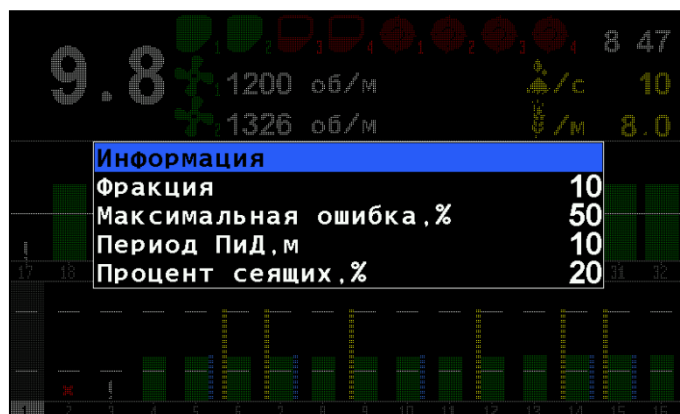
Рисунок 10 Параметры датчика высева
