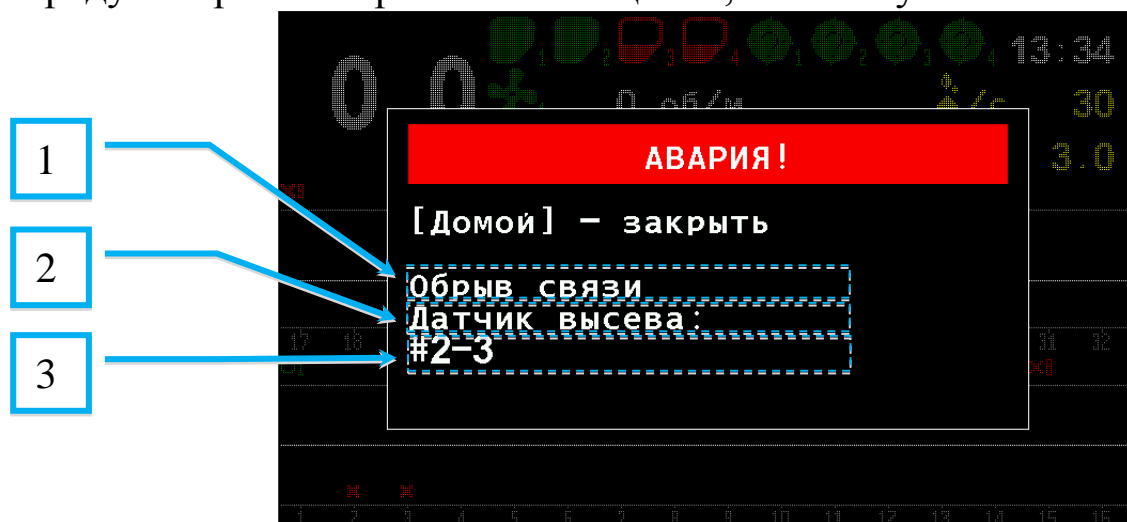
Рисунок 7 Аварийное сообщение
