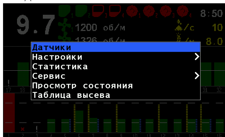
Рисунок 12 Главное меню
